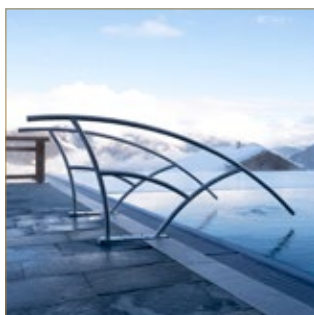
Main courante L 2400 · Ø 42,4 · H 880 mm
