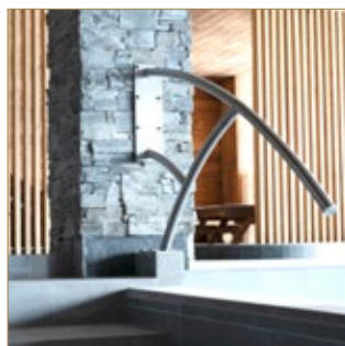
Main courante murale L 1710 · Ø 42,4 · H 880 mm
